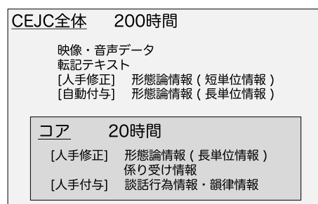
図 2.1: CEJC の構成
