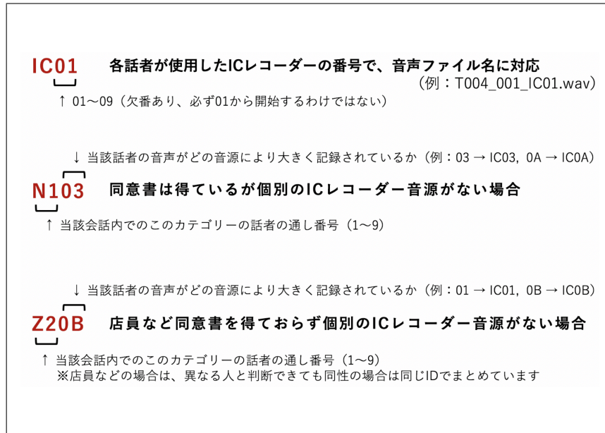
図 2.5: 話者ラベル
